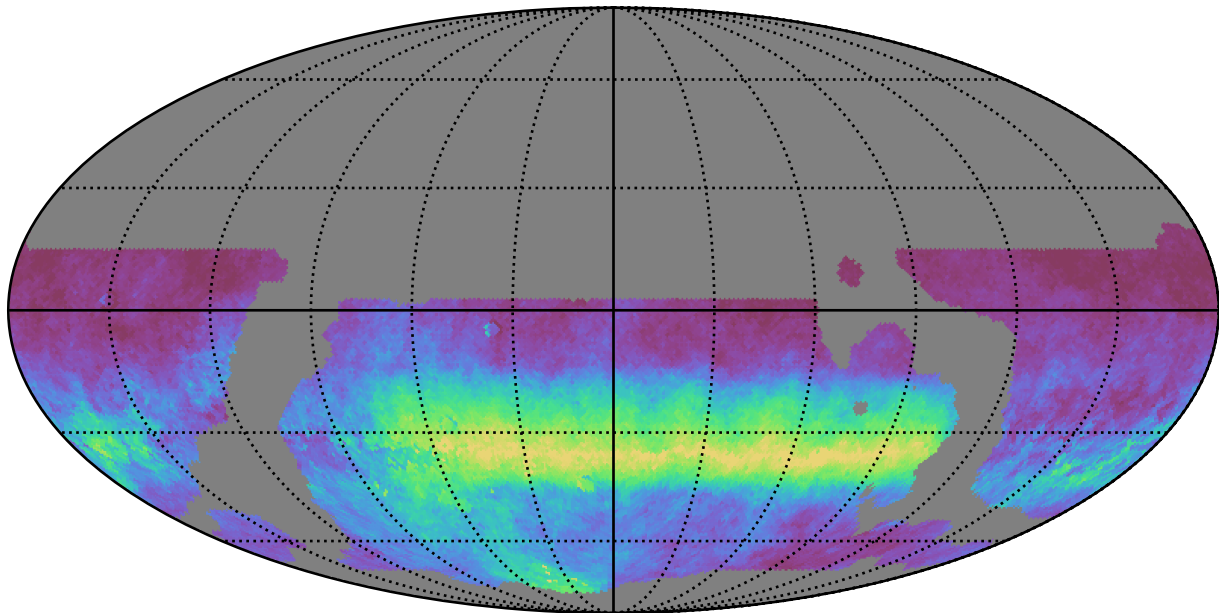
weather_cloudso20v3.4_10yrs WFD r band: AngleRms rotSkyPos
