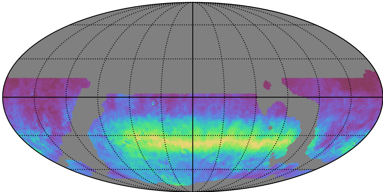
weather_cloudso20v3.4_10yrs WFD i band: AngleRms rotSkyPos
