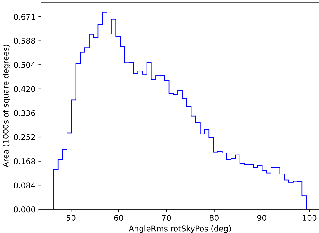
weather_cloudso20v3.4_10yrs WFD i band: AngleRms rotSkyPos
