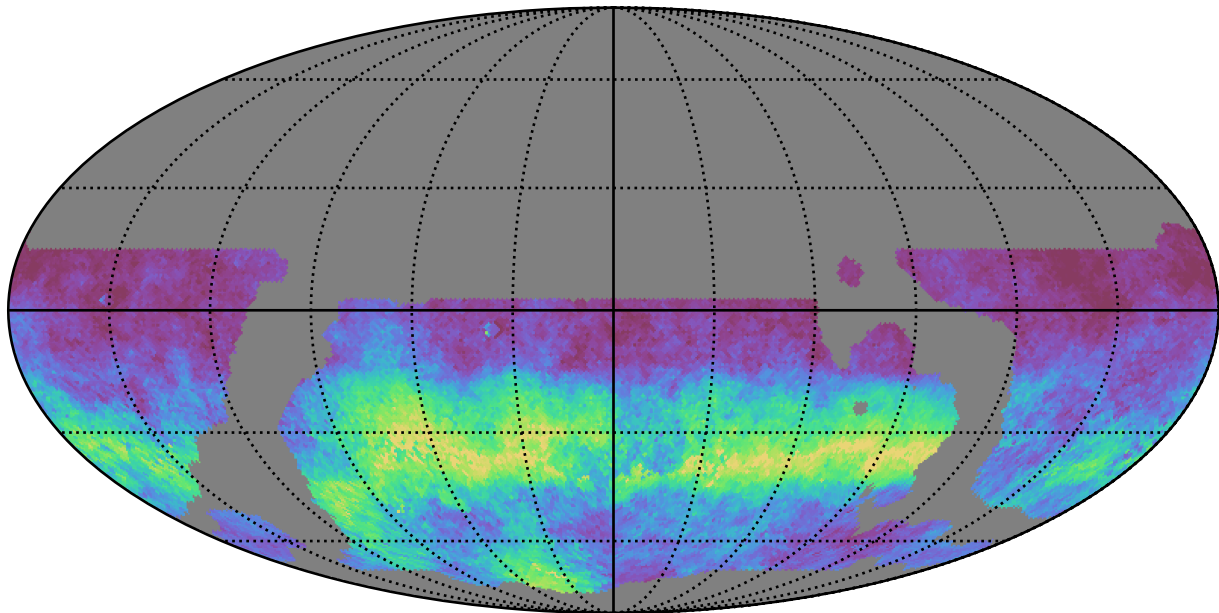
weather_cloudso20v3.4_10yrs WFD g band: AngleRms rotSkyPos
