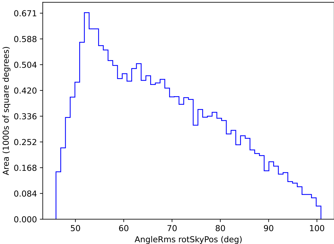
weather_cloudso20v3.4_10yrs WFD g band: AngleRms rotSkyPos
