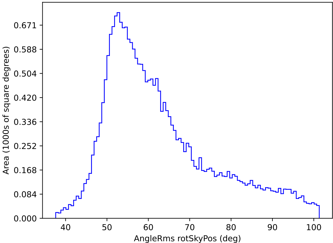
weather_cloudso20v3.4_10yrs All sky y band: AngleRms rotSkyPos
