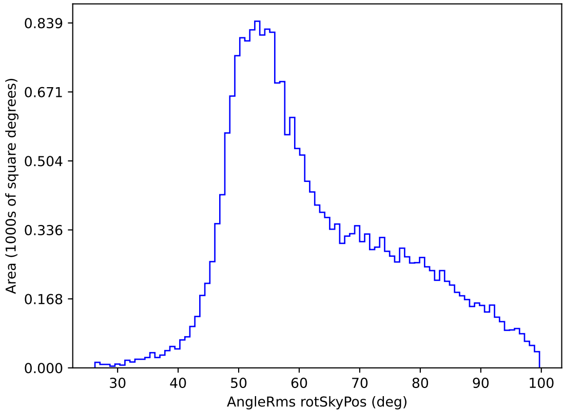
weather_cloudso20v3.4_10yrs All sky u band: AngleRms rotSkyPos
