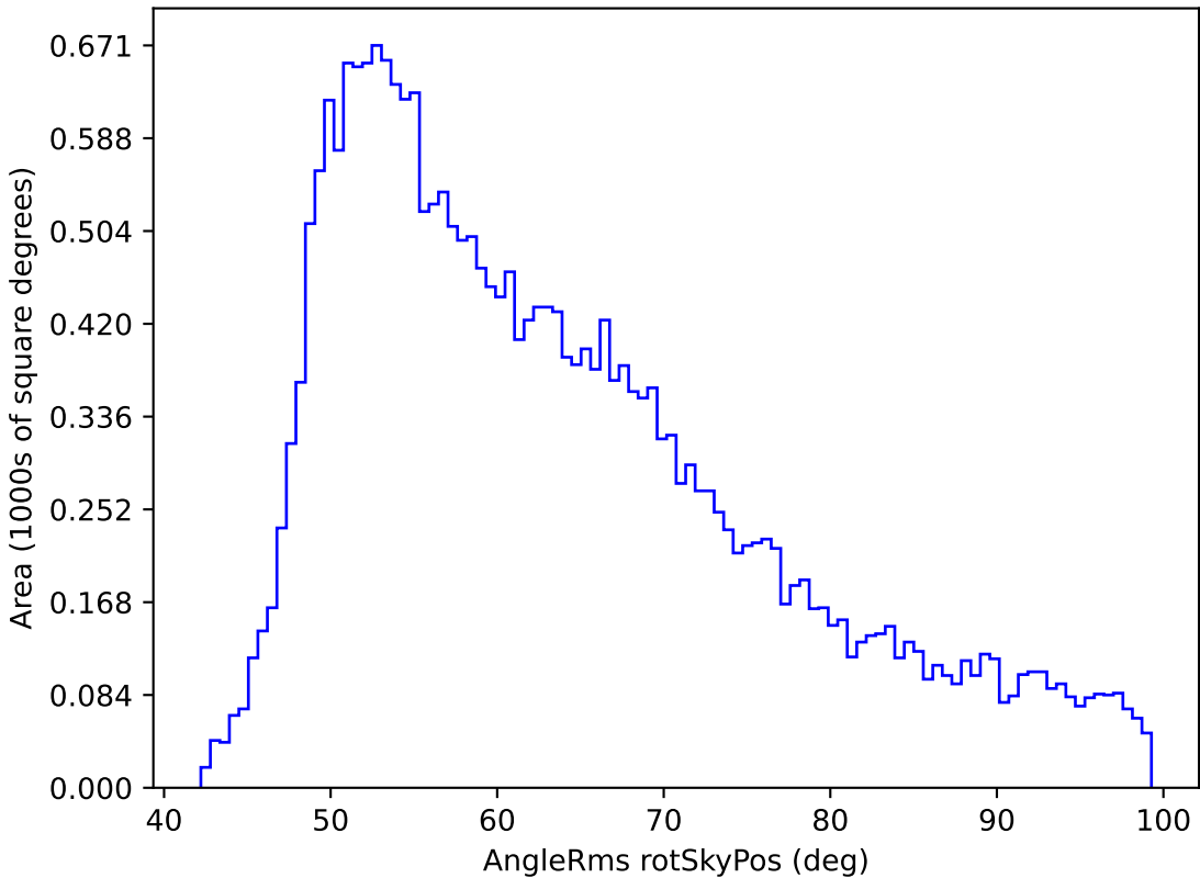
weather_cloudso20v3.4_10yrs All sky r band: AngleRms rotSkyPos
