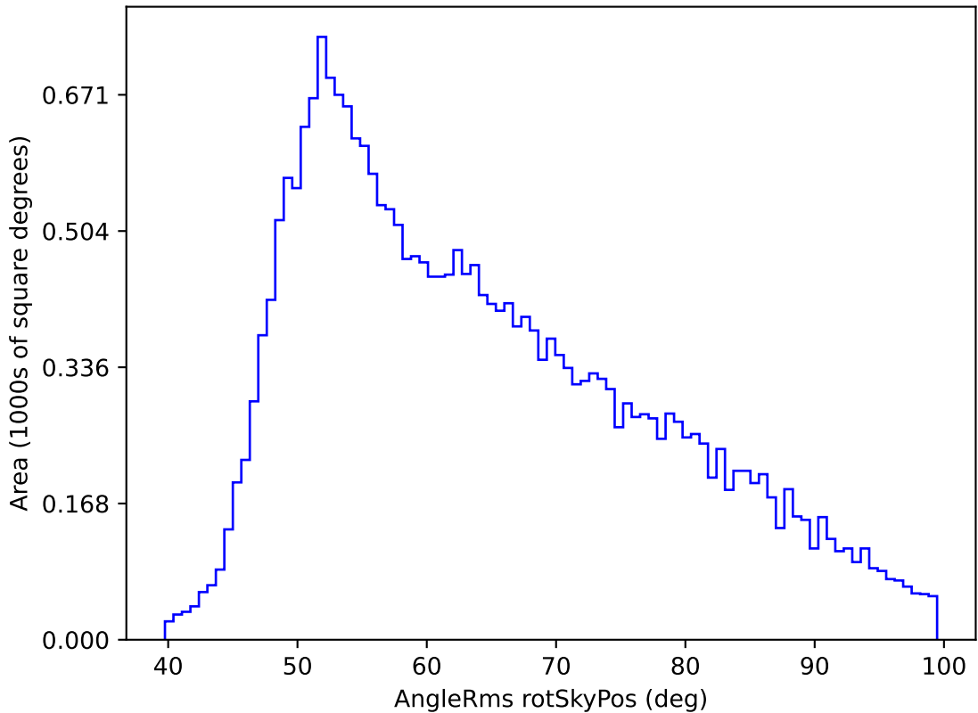
weather_cloudso20v3.4_10yrs All sky g band: AngleRms rotSkyPos
