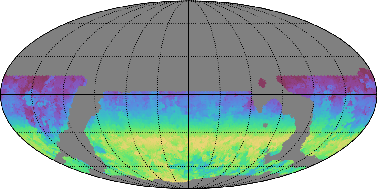
weather_cloudso20v3.4_10yrs WFD z band: AngleRange rotSkyPos
