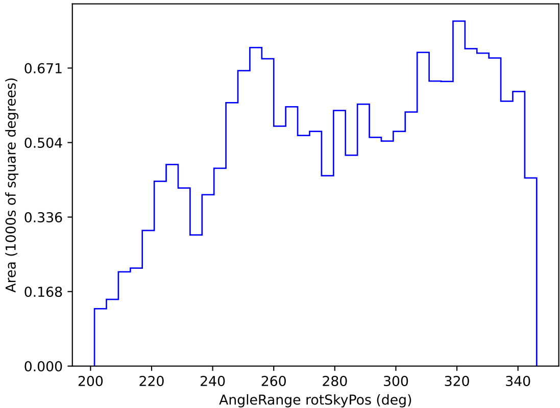
weather_cloudso20v3.4_10yrs WFD z band: AngleRange rotSkyPos
