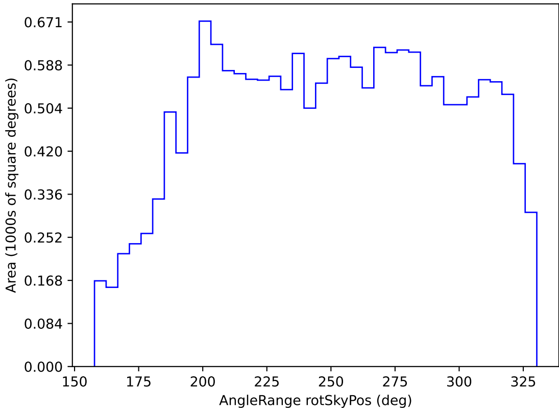
weather_cloudso20v3.4_10yrs WFD u band: AngleRange rotSkyPos
