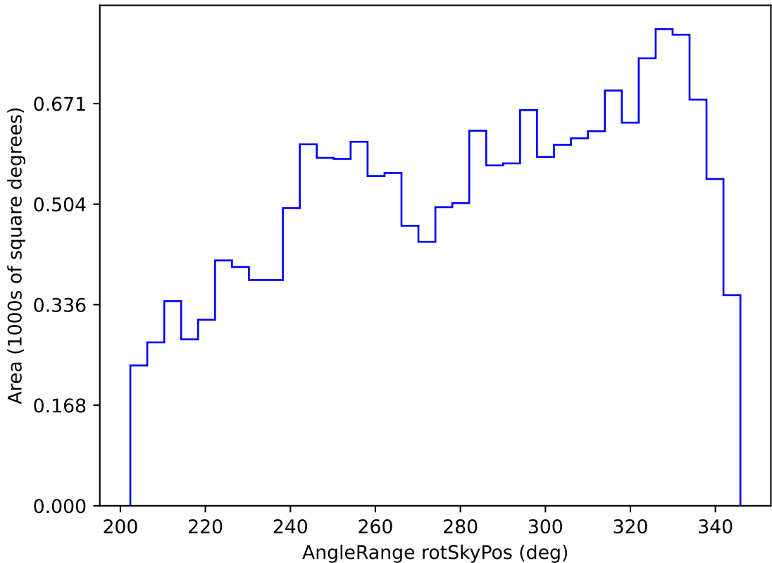
weather_cloudso20v3.4_10yrs WFD r band: AngleRange rotSkyPos
