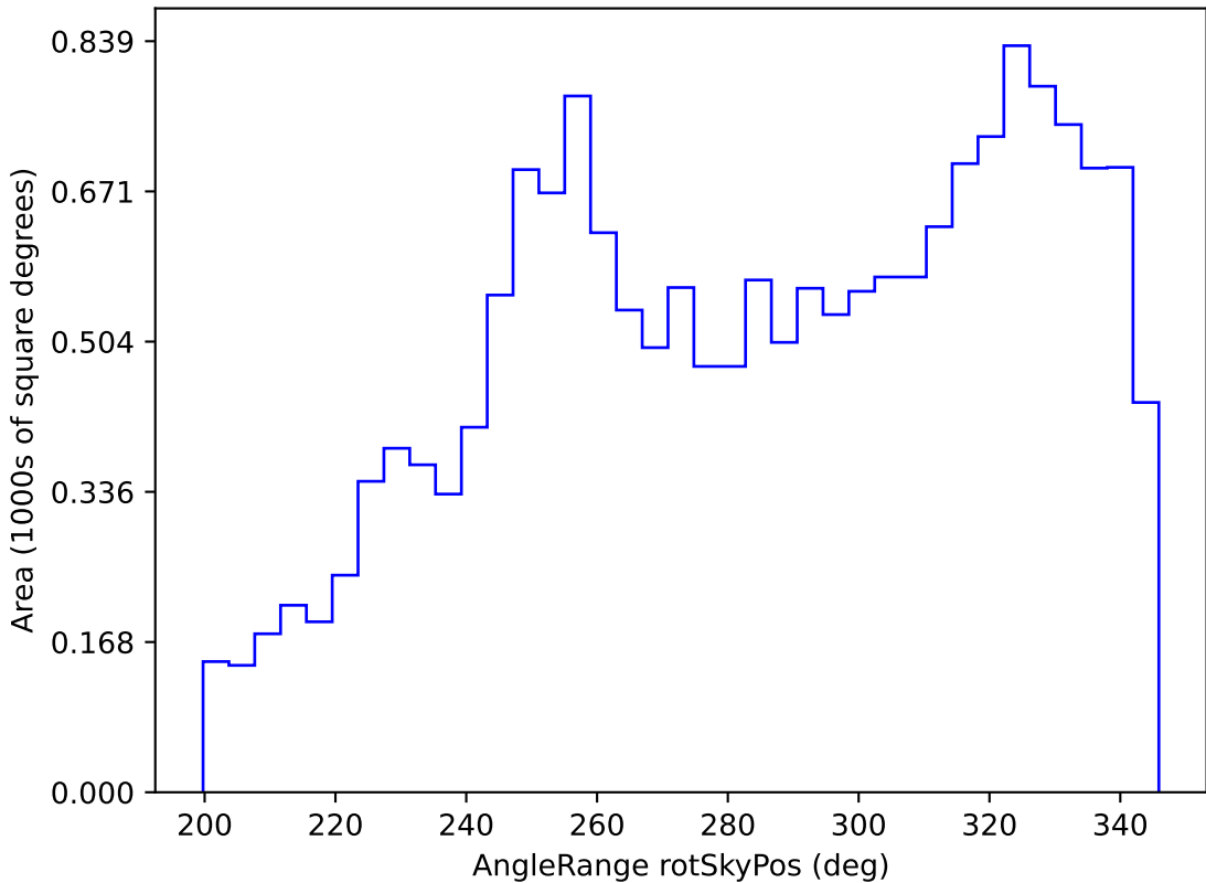
weather_cloudso20v3.4_10yrs WFD i band: AngleRange rotSkyPos
