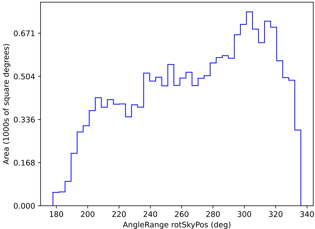
weather_cloudso20v3.4_10yrs WFD g band: AngleRange rotSkyPos
