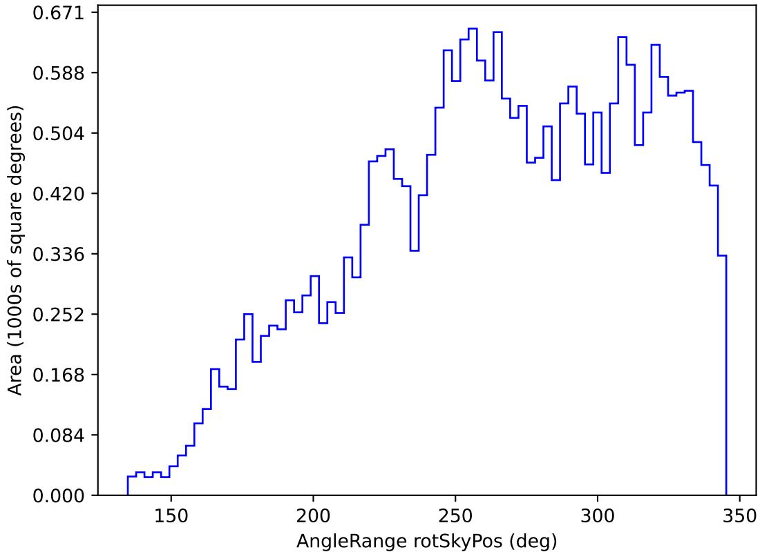
weather_cloudso20v3.4_10yrs All sky z band: AngleRange rotSkyPos
