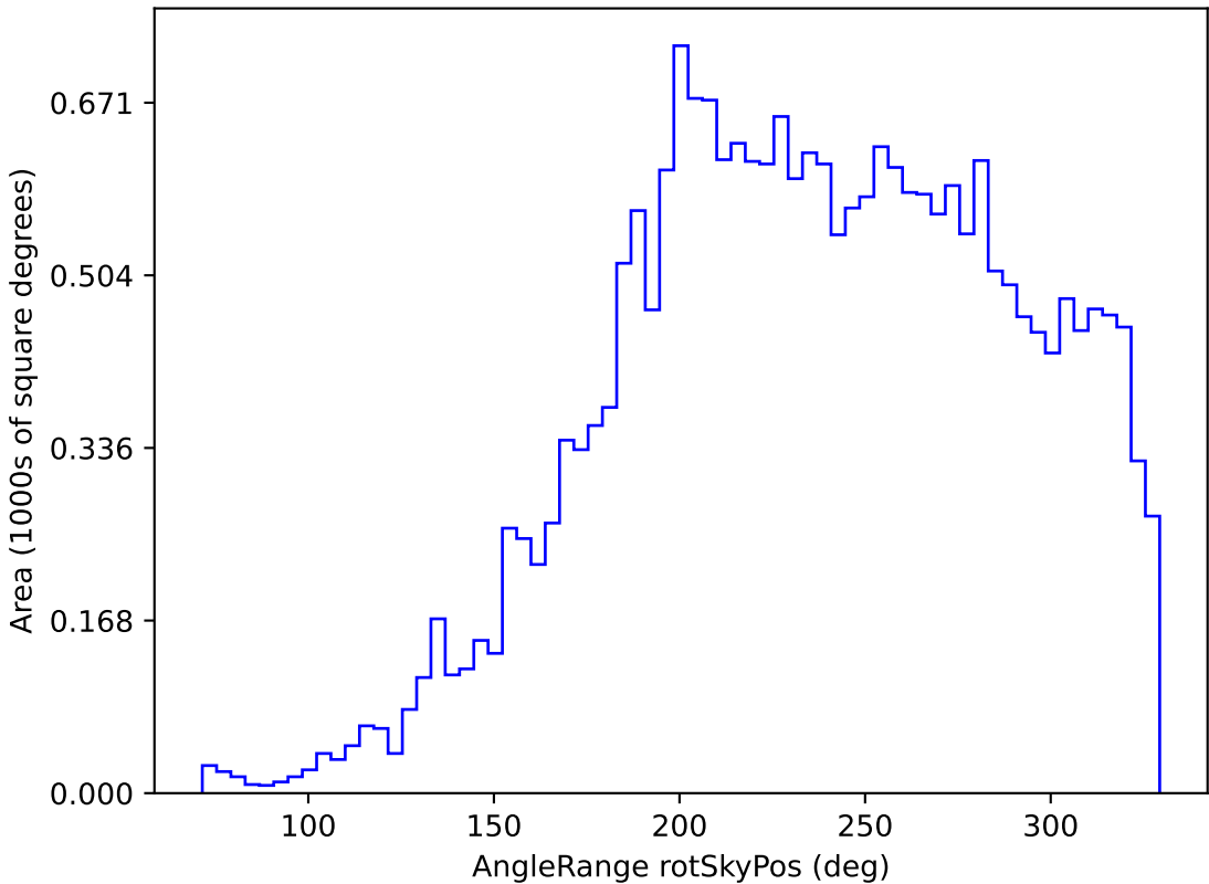
weather_cloudso20v3.4_10yrs All sky u band: AngleRange rotSkyPos
