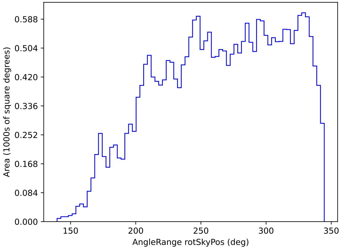
weather_cloudso20v3.4_10yrs All sky r band: AngleRange rotSkyPos
