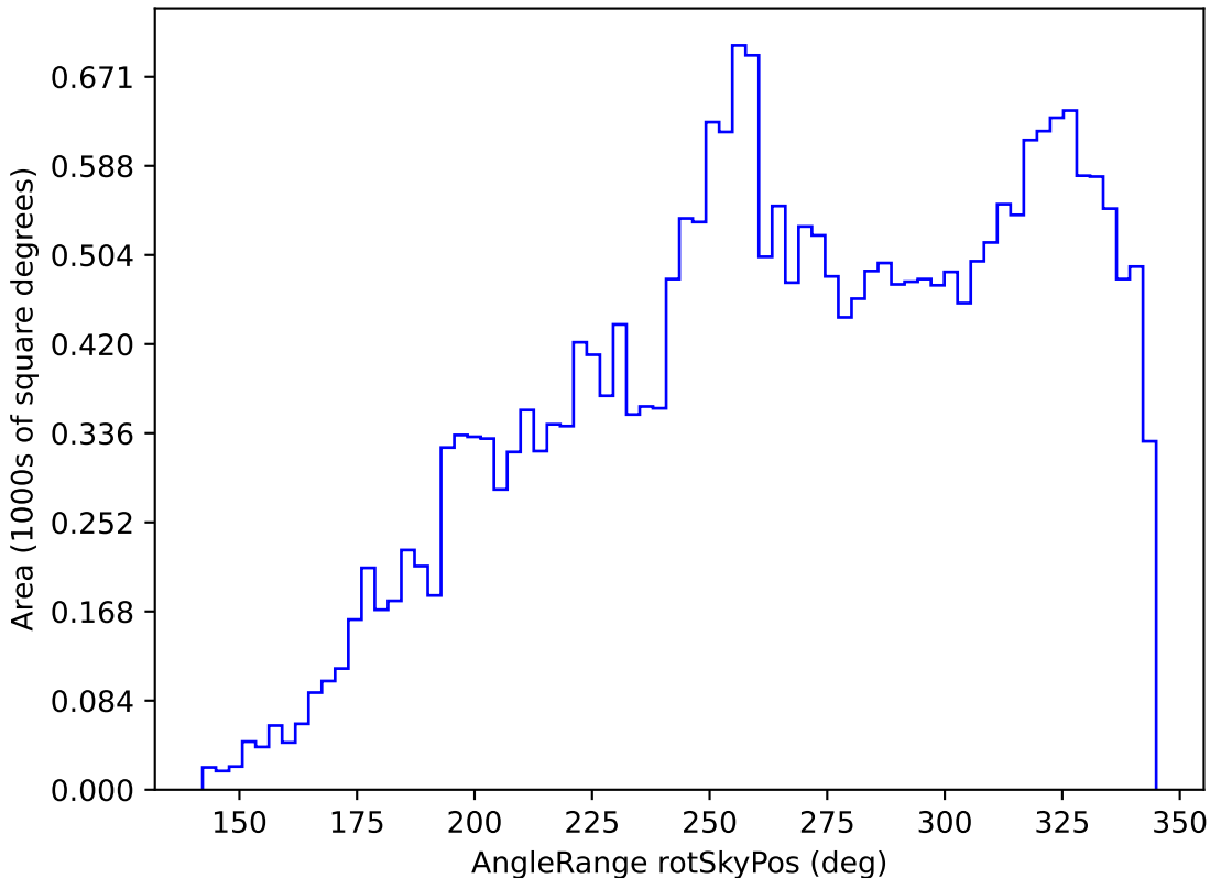
weather_cloudso20v3.4_10yrs All sky i band: AngleRange rotSkyPos
