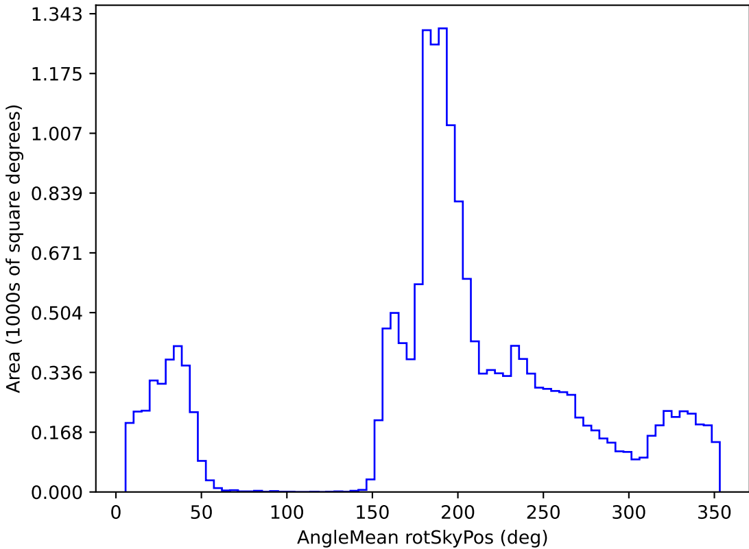
weather_cloudso20v3.4_10yrs WFD z band: AngleMean rotSkyPos
