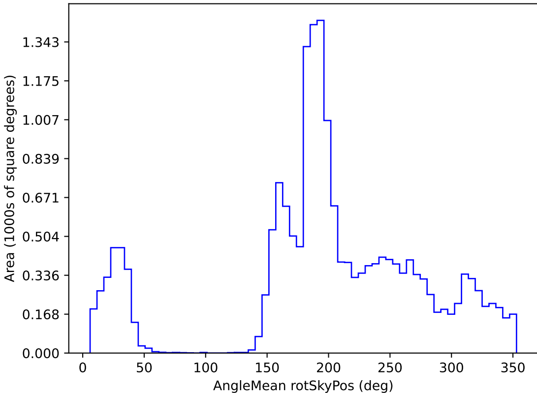
weather_cloudso20v3.4_10yrs WFD y band: AngleMean rotSkyPos
