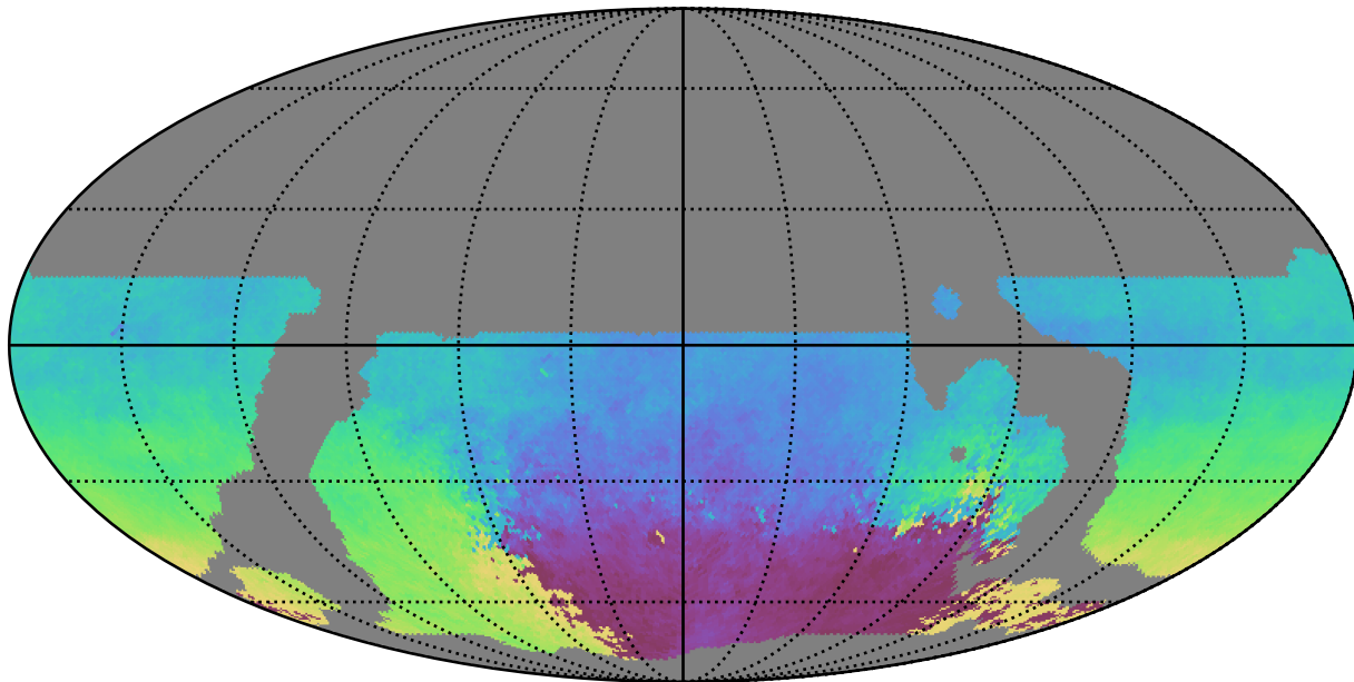
weather_cloudso20v3.4_10yrs WFD u band: AngleMean rotSkyPos
