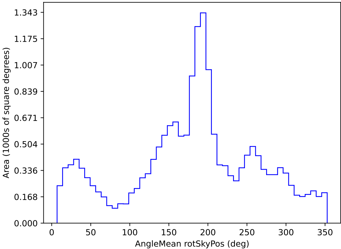
weather_cloudso20v3.4_10yrs WFD u band: AngleMean rotSkyPos
