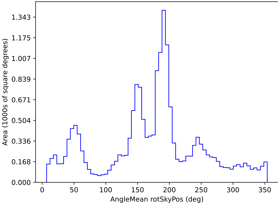
weather_cloudso20v3.4_10yrs WFD g band: AngleMean rotSkyPos
