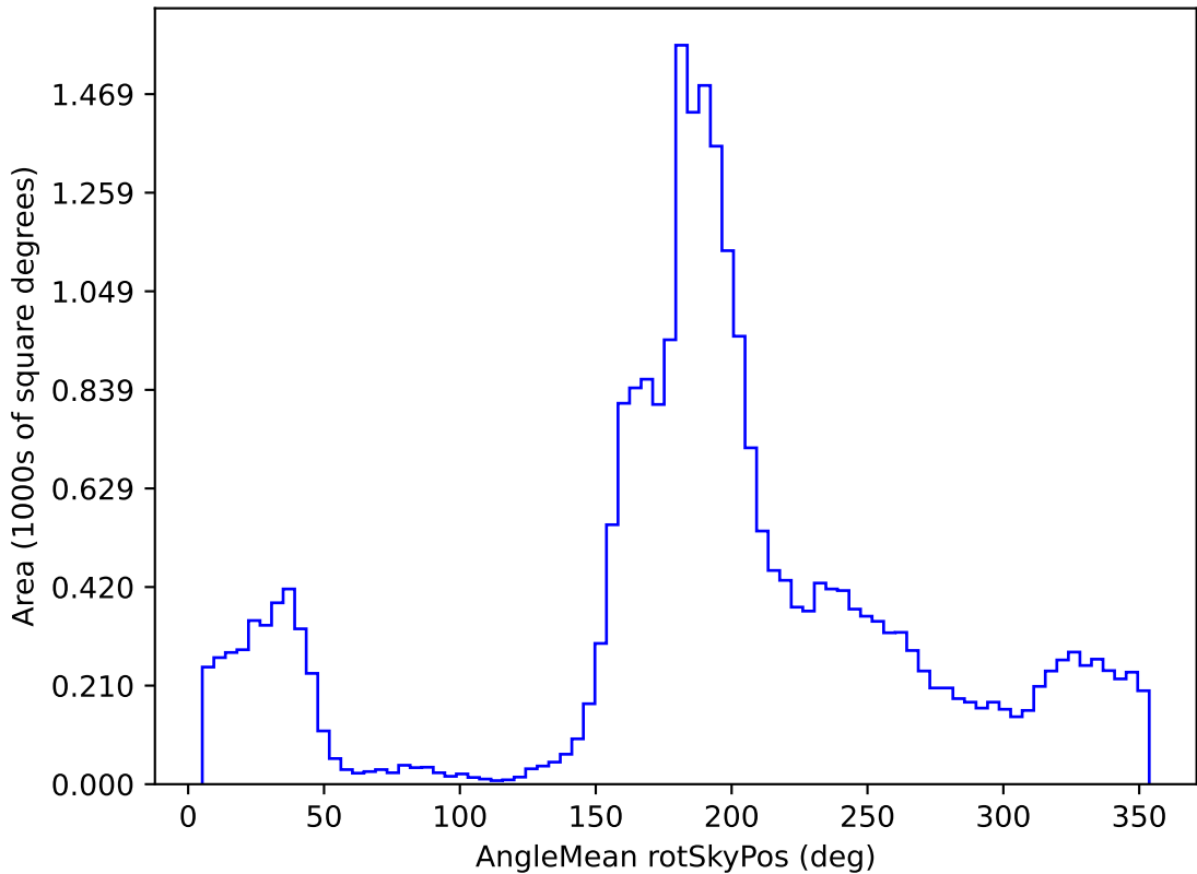
weather_cloudso20v3.4_10yrs All sky z band: AngleMean rotSkyPos
