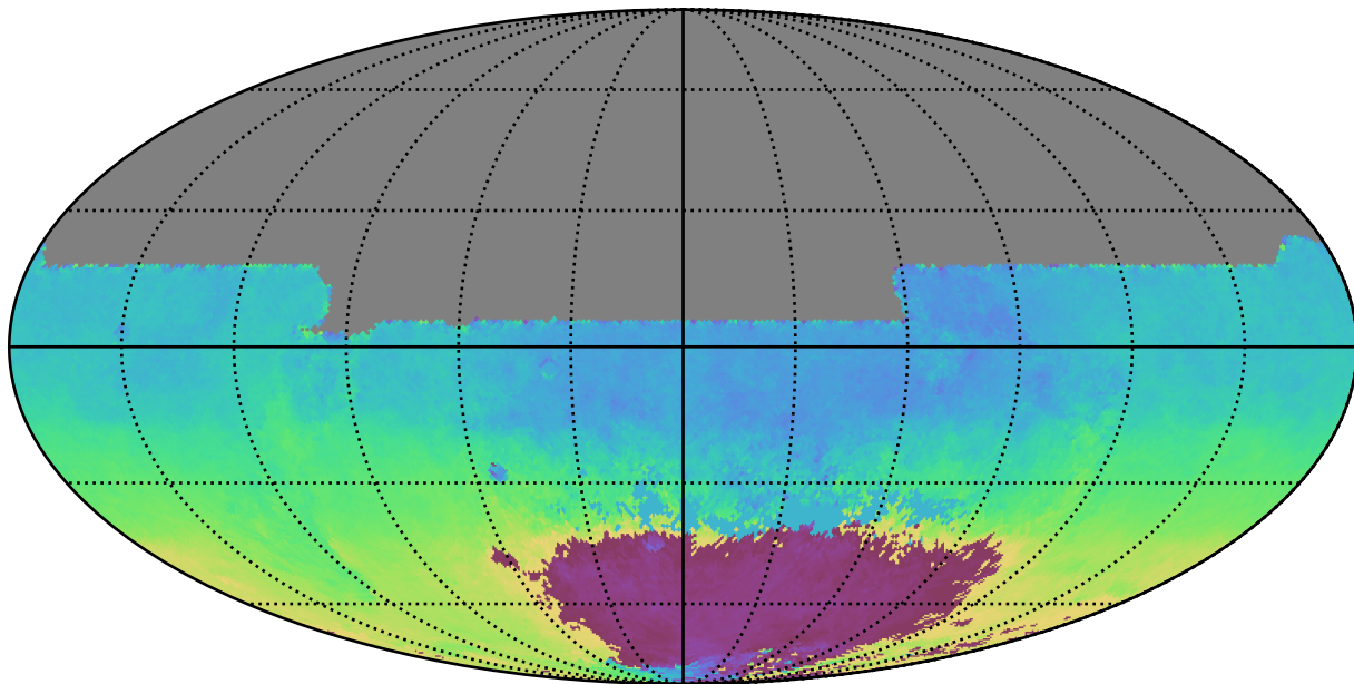
weather_cloudso20v3.4_10yrs All sky y band: AngleMean rotSkyPos
