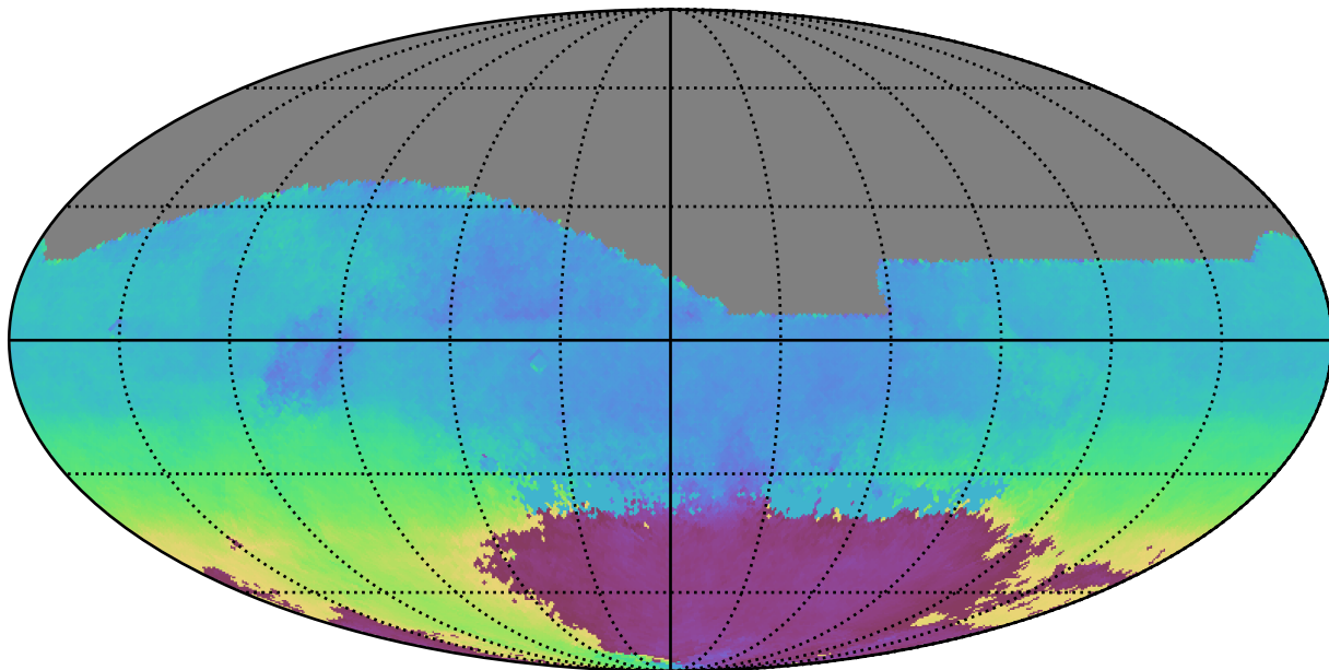
weather_cloudso20v3.4_10yrs All sky r band: AngleMean rotSkyPos
