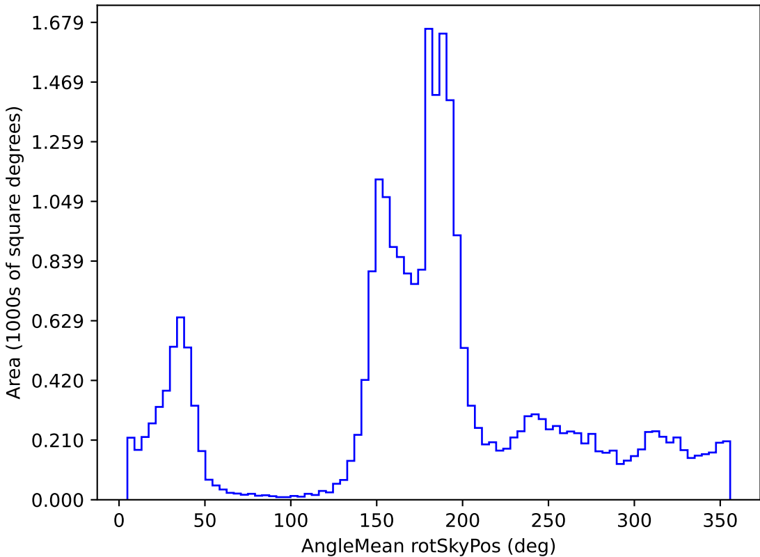
weather_cloudso20v3.4_10yrs All sky r band: AngleMean rotSkyPos
