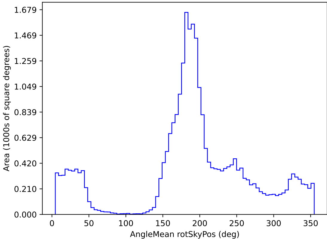
weather_cloudso20v3.4_10yrs All sky i band: AngleMean rotSkyPos
