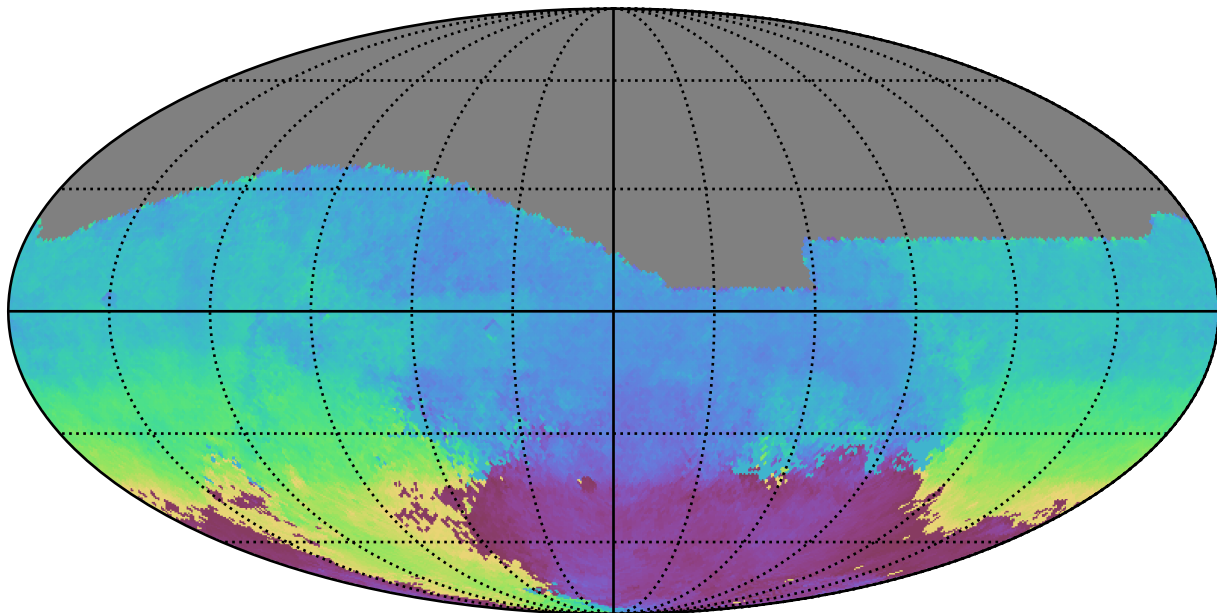
weather_cloudso20v3.4_10yrs All sky g band: AngleMean rotSkyPos
