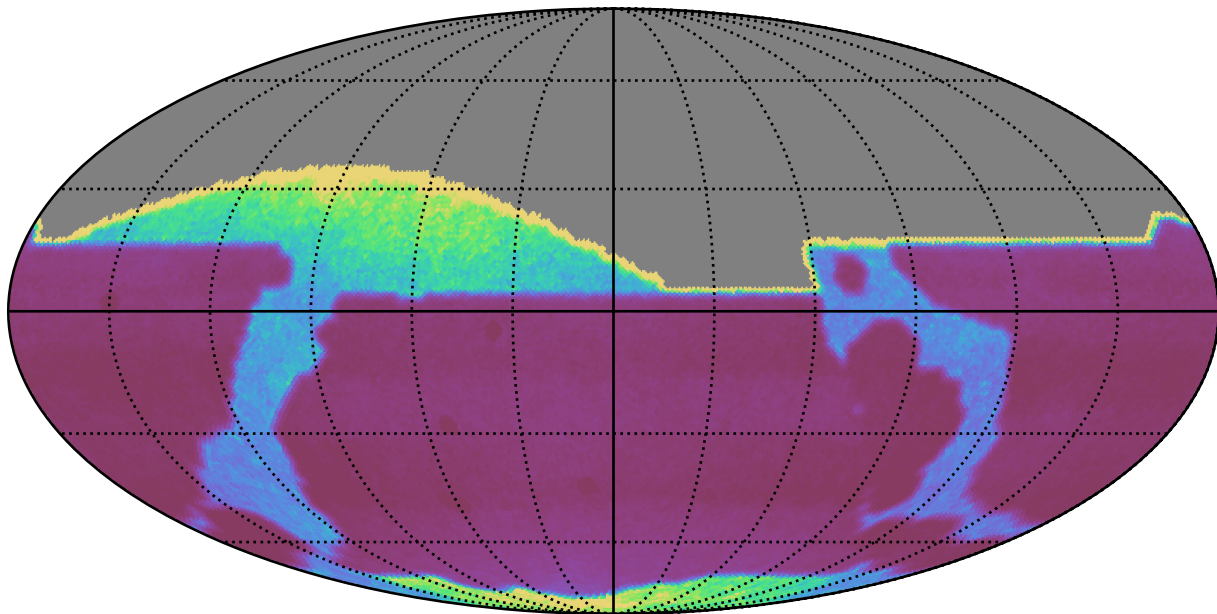
weather_cloudso20v3.4_10yrs : properMotion
