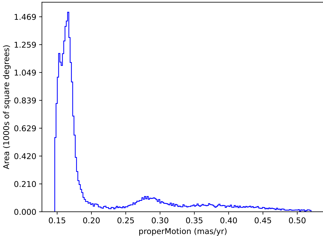
weather_cloudso20v3.4_10yrs : properMotion
