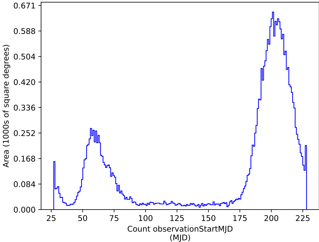
weather_cloudso20v3.4_10yrs i: Count observationStartMJD
