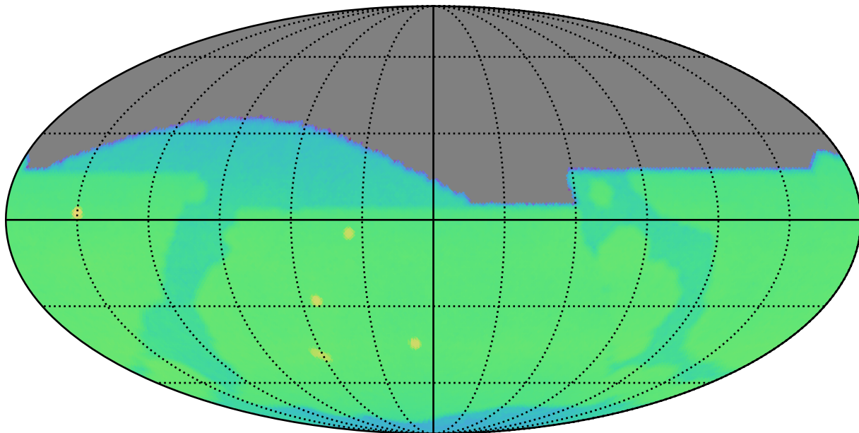
weather_cloudso20v3.4_10yrs r: CoaddM5
