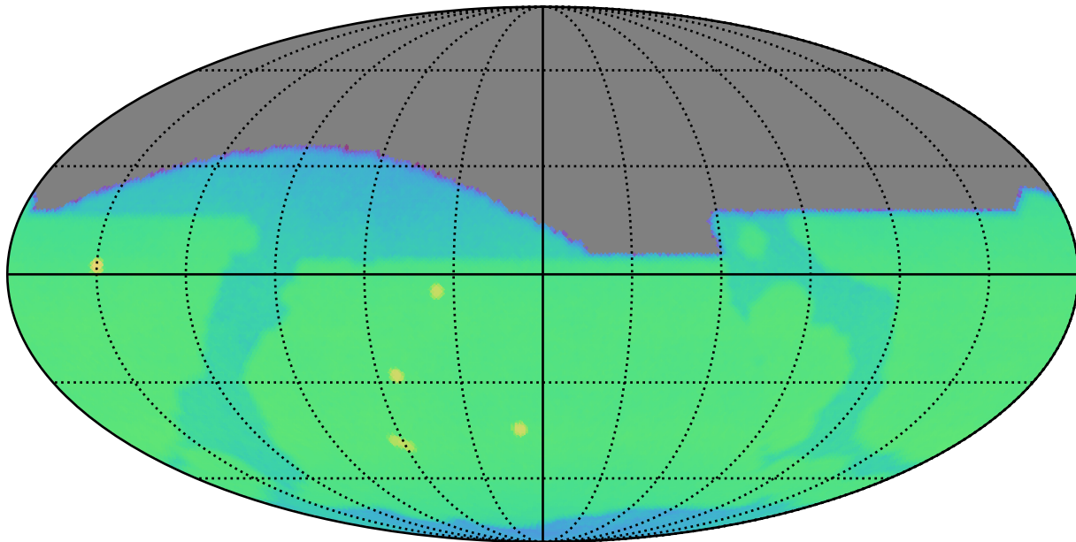
weather_cloudso20v3.4_10yrs i: CoaddM5
