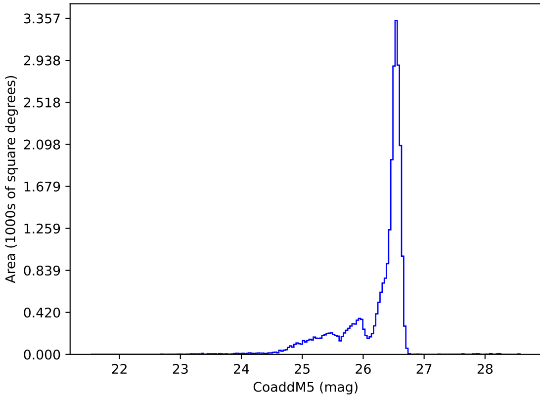
weather_cloudso20v3.4_10yrs i: CoaddM5
