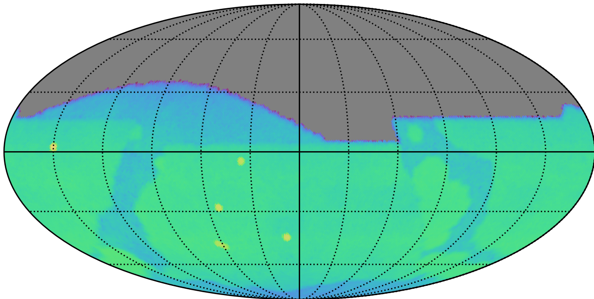
weather_cloudso20v3.4_10yrs g: CoaddM5
