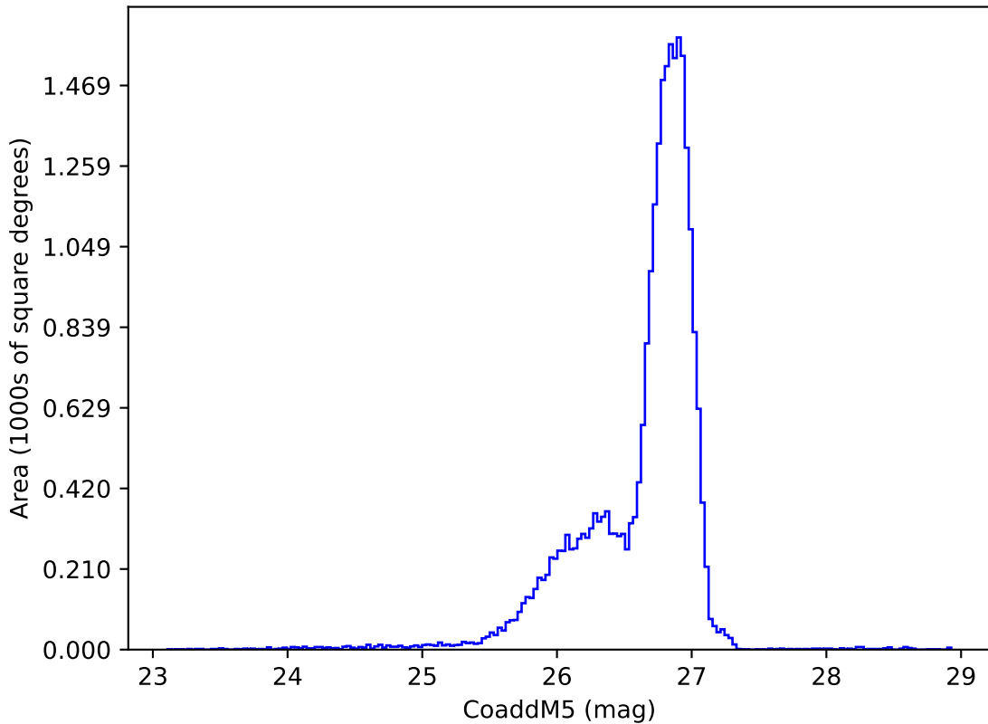
weather_cloudso20v3.4_10yrs g: CoaddM5
