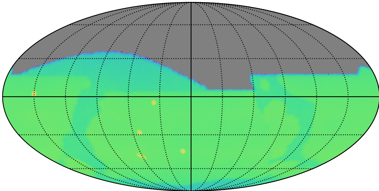
weather_cloudso20v3.4_10yrs : CoaddM5
