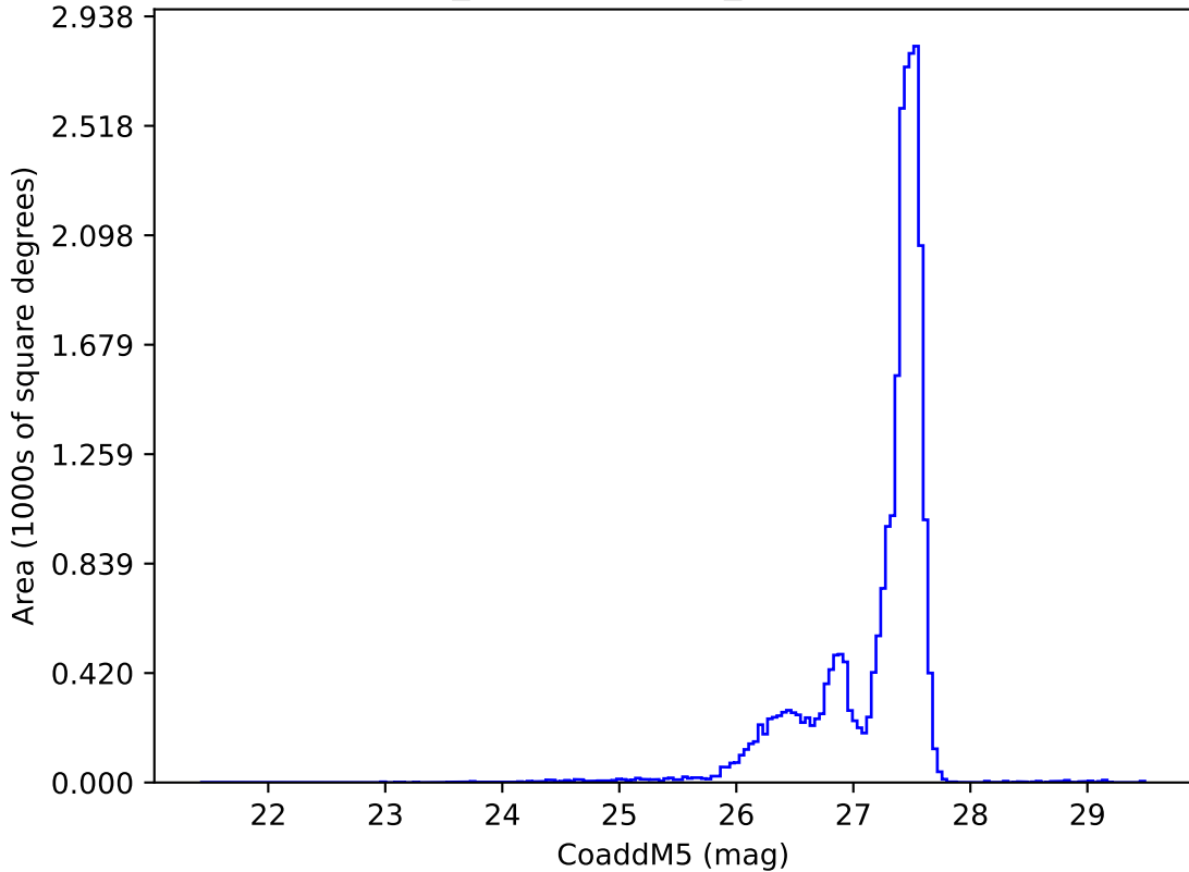
weather_cloudso20v3.4_10yrs : CoaddM5
