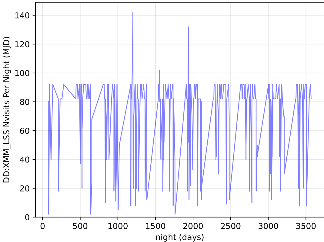
weather_cloudso20v3.4_10yrs all bands: DD:XMM_LSS Nvisits Per Night
