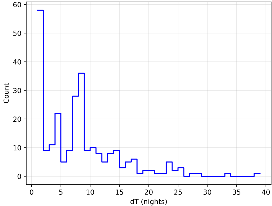
weather_cloudso20v3.4_10yrs all bands: DD:XMM_LSS Delta Nights Histogram
