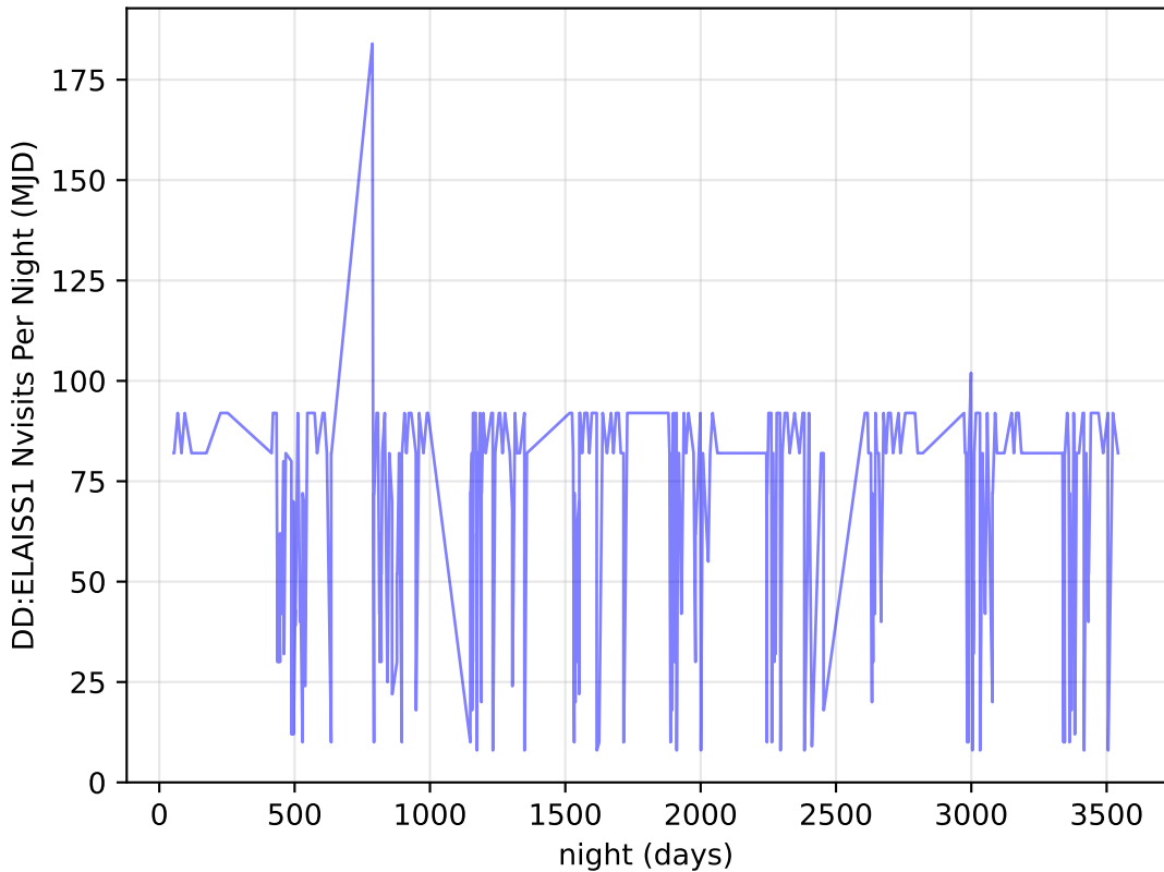
weather_cloudso20v3.4_10yrs all bands: DD:ELAISS1 Nvisits Per Night
