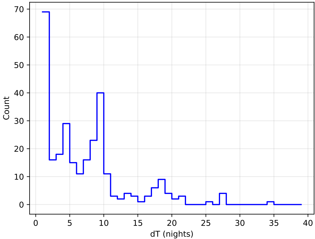
weather_cloudso20v3.4_10yrs all bands: DD:ELAISS1 Delta Nights Histogram
