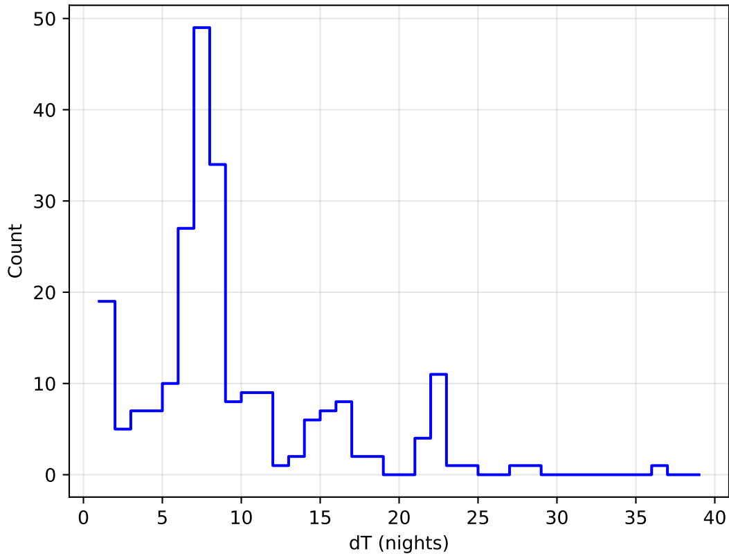
weather_cloudso20v3.4_10yrs all bands: DD:EDFS Delta Nights Histogram
