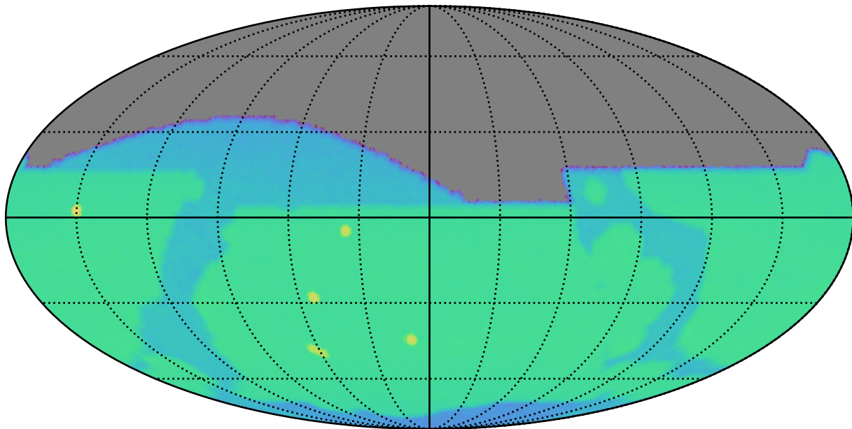
weather_cloudso1v3.4_10yrs i: SurfaceBrightLimit
