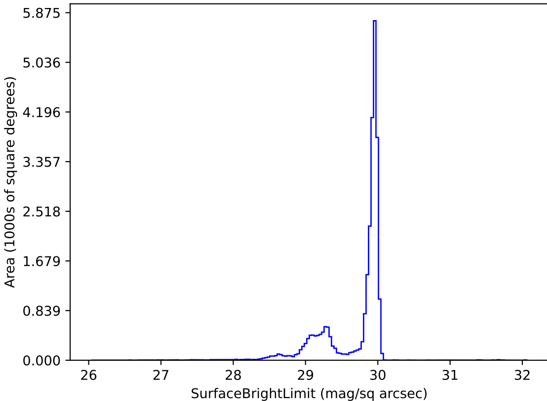
weather_cloudso1v3.4_10yrs i: SurfaceBrightLimit
