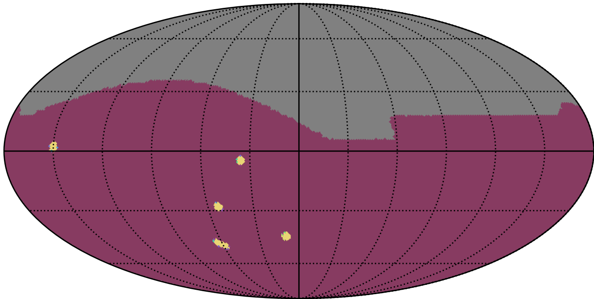
weather_cloudso1v3.4_10yrs : NumberOfQuickRevisits
