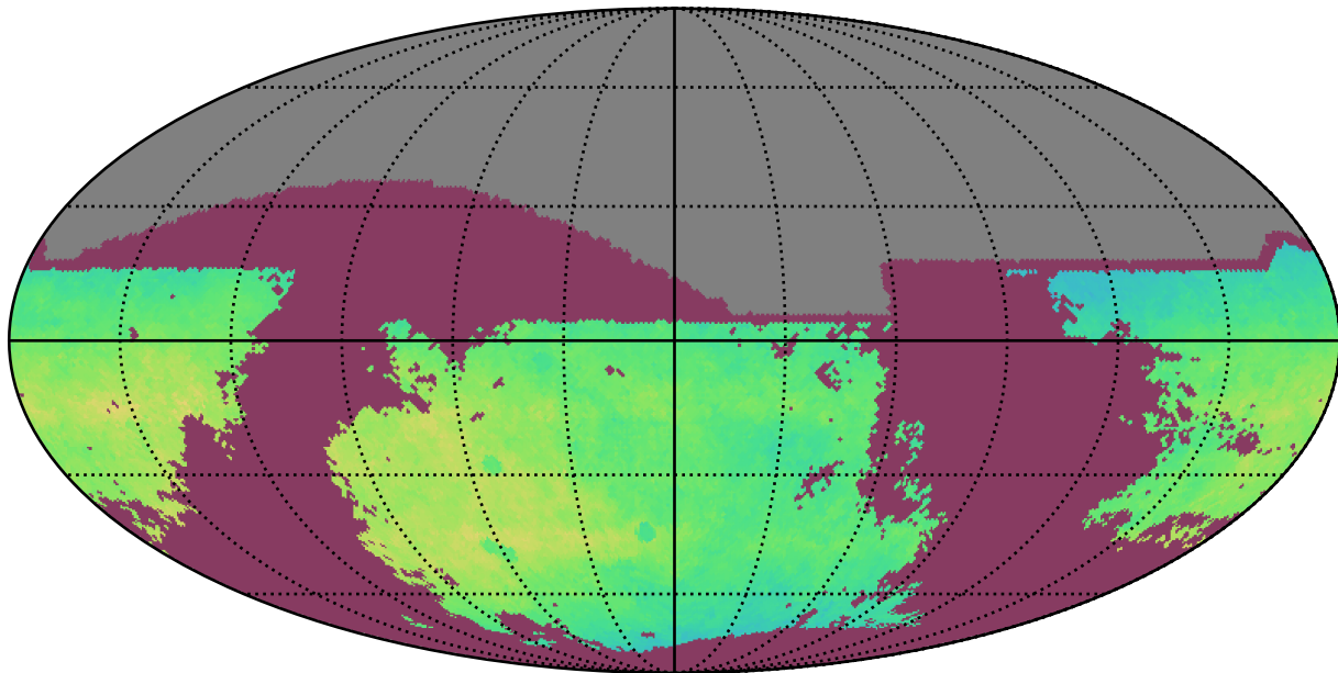
weather_cloudso1v3.4_10yrs i: NgalScale
