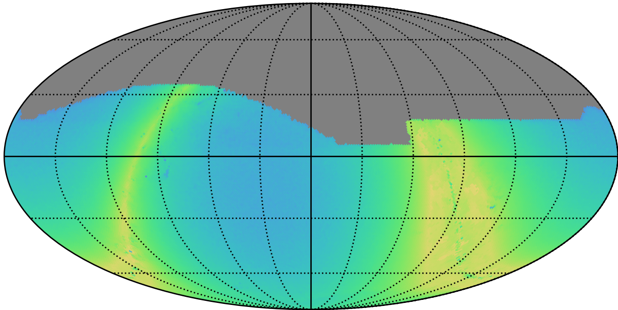
weather_cloudso1v3.4_10yrs i: N stars to Precision 0.20
